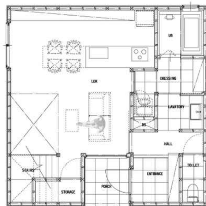
2階建 延床面積/102.53㎡
